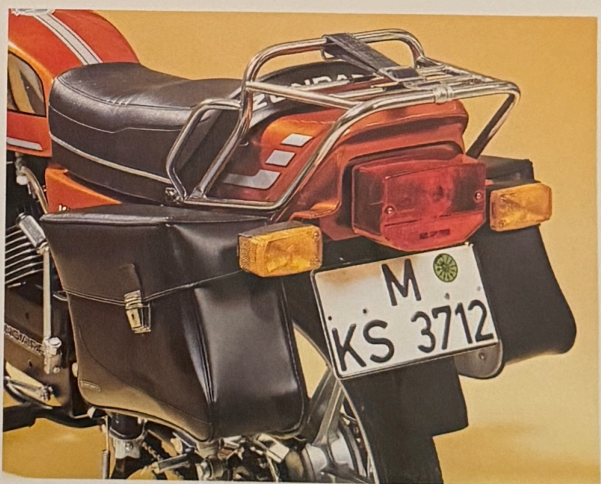
Verchromter Packtaschenträger , einteilig. Für Mokick- und Leichtkraftrad-Typen 529 und 530 mit Spoiler-Gepäckträger (bis einschl. Baujahr 1980). Bestell-Nr. 530-21.605
